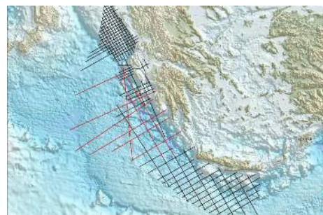
Ο χάρτης με τις διελεύσεις του νορβηγικού ερευνητικού από τα σημεία όπου εικάζεται ότι υπάρχουν υδρογονάνθρακες στο Ιόνιο και νότια της Κρήτης.
